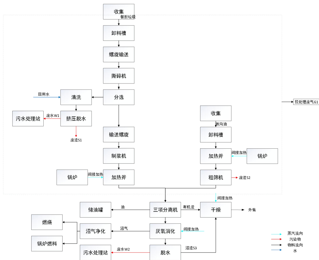
图 3.5-2 主体工艺流程及产污节点图
