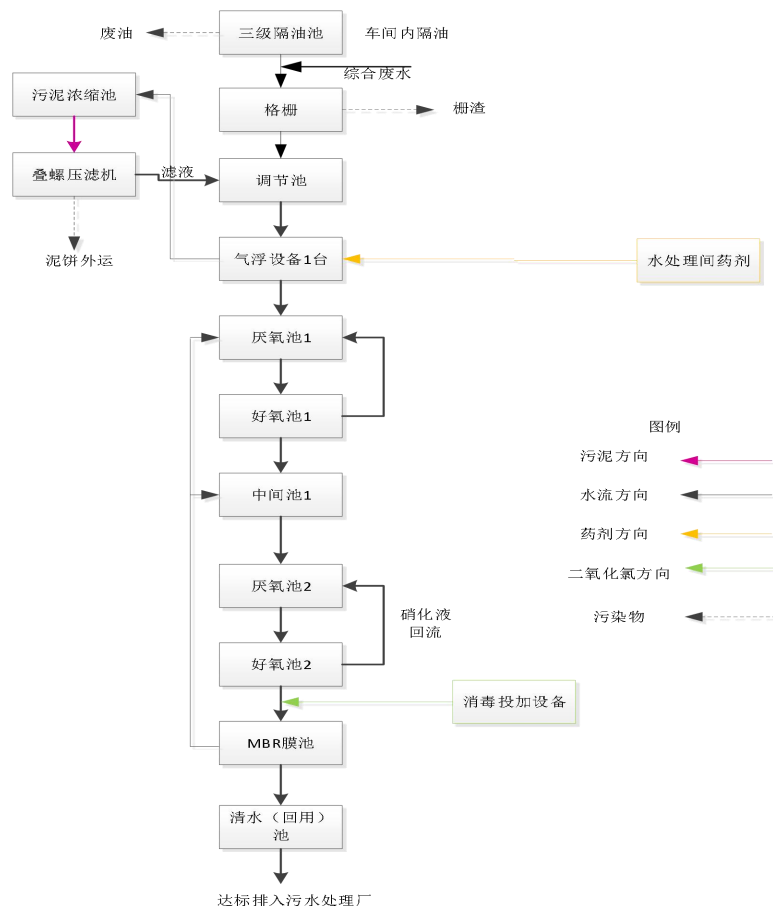
图 3.5-4 污水处理站工艺流程图
